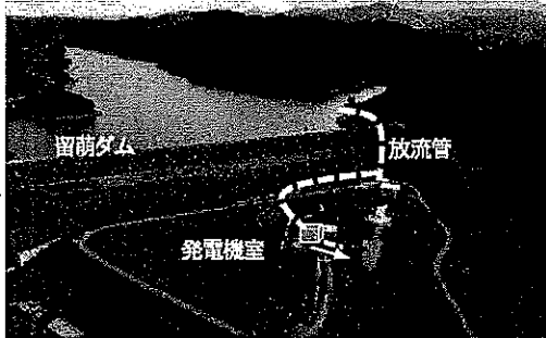
未利用の河川維持放流水を活用した小水力発電の例 (留萌ダム (留萌市))
